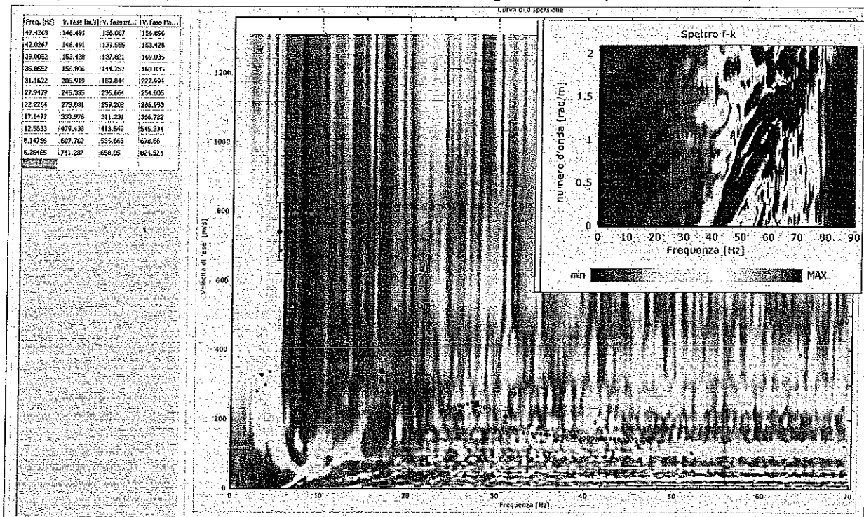
Figura 3: Curva di dispersione e spettro f-k
